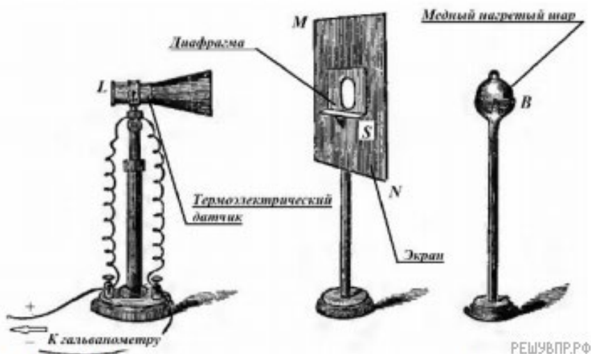
Рис. 1. Исследование прозрачности твёрдых тел
