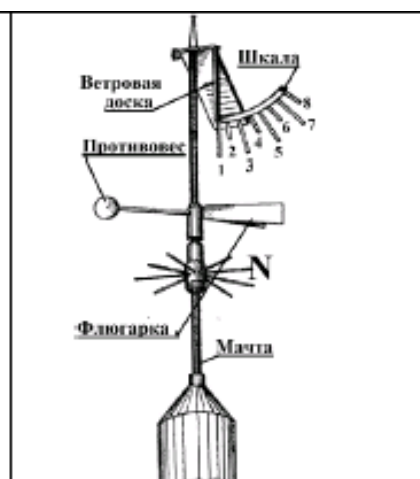
Рис. 2. Флюгер-анемометр Вильда
