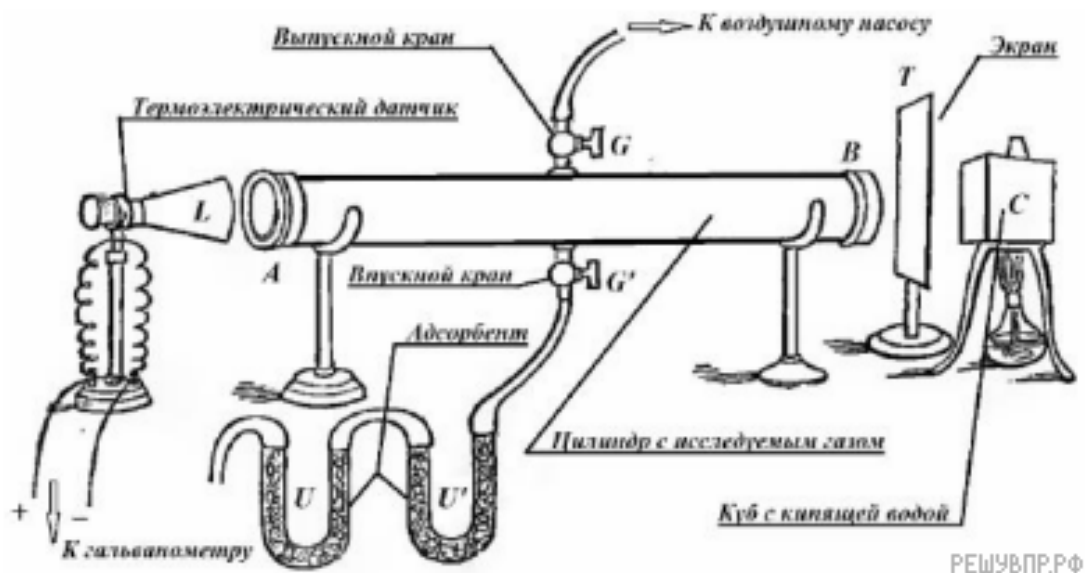
Рис. 2. Исследование прозрачности газов
