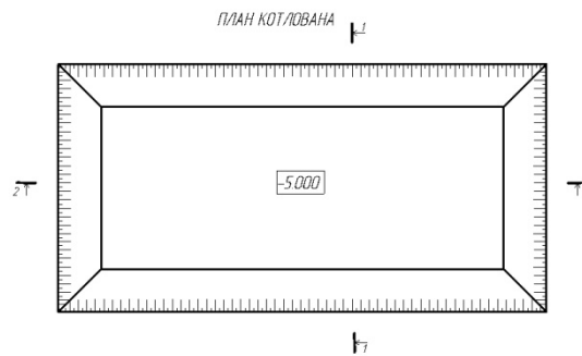
рис.5 план котлована
