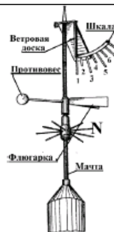
Рис. 2. Флюгер-анемометр Вильда
