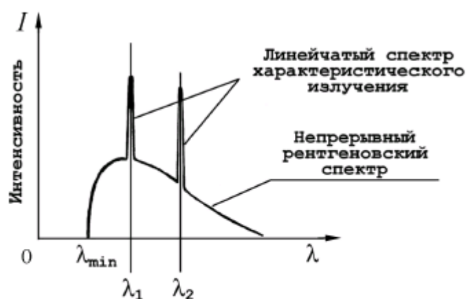
Рис. 2б. Рентгеновский спектр (тормозной и характеристический)
